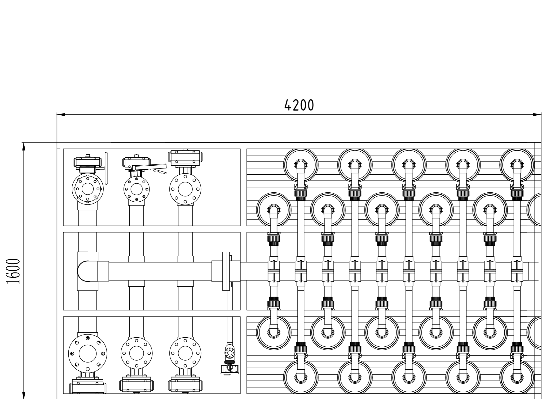
Вид сверху
