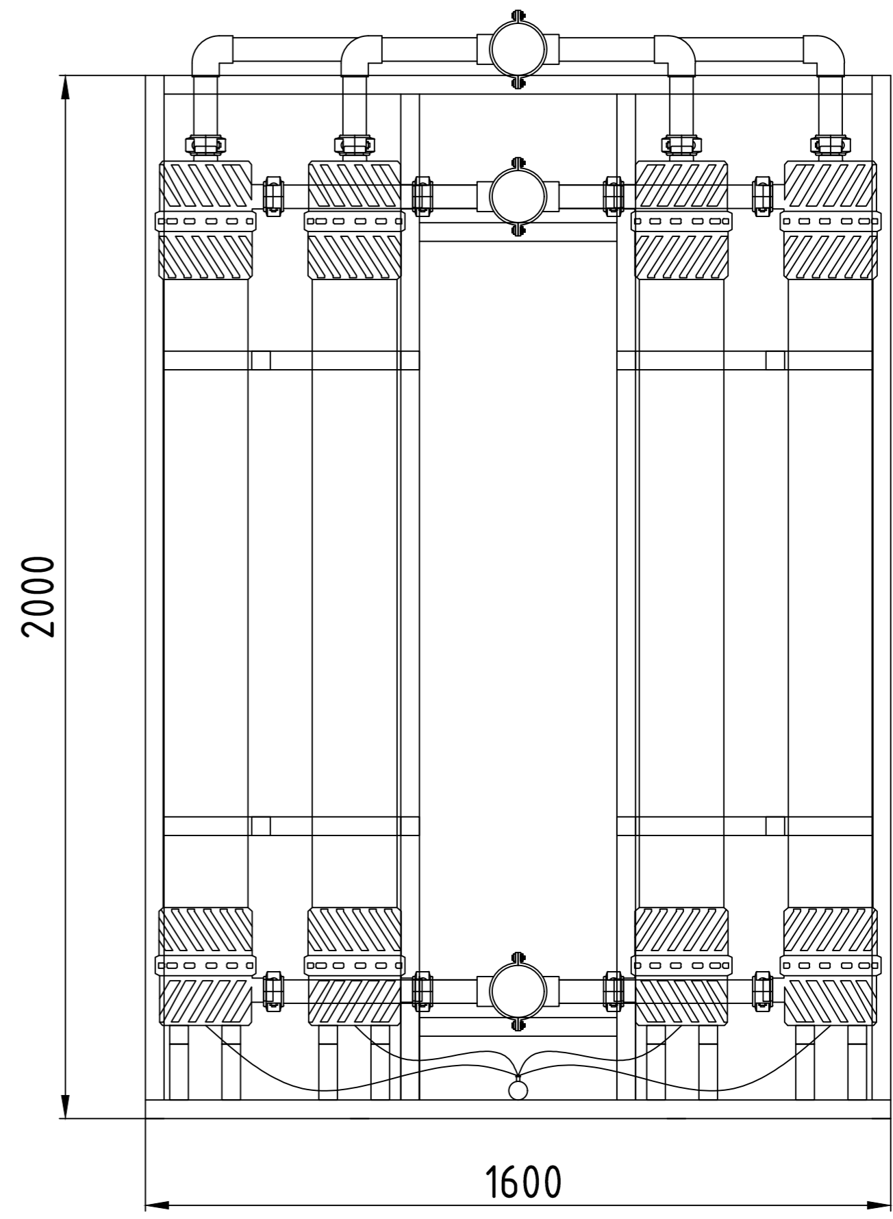
Вид слева
