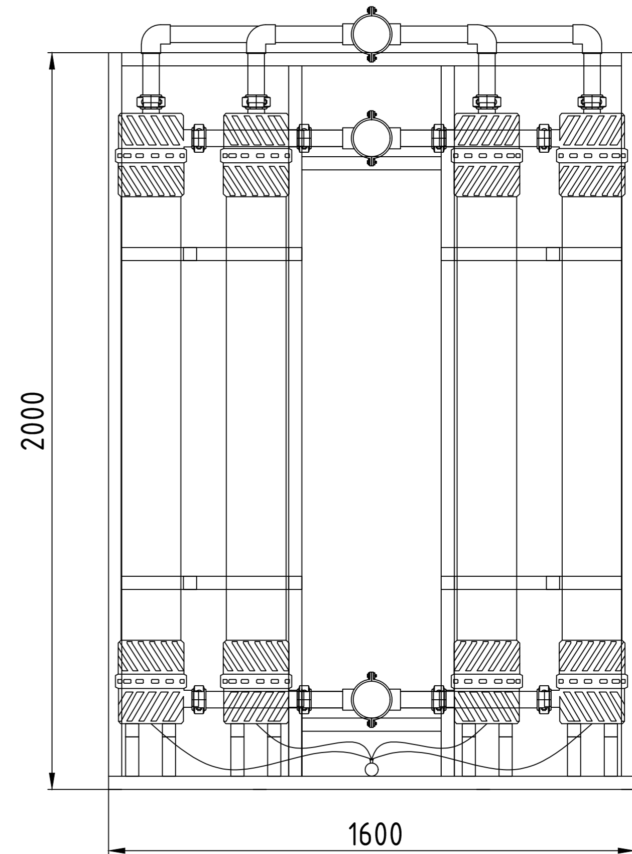
Вид слева
