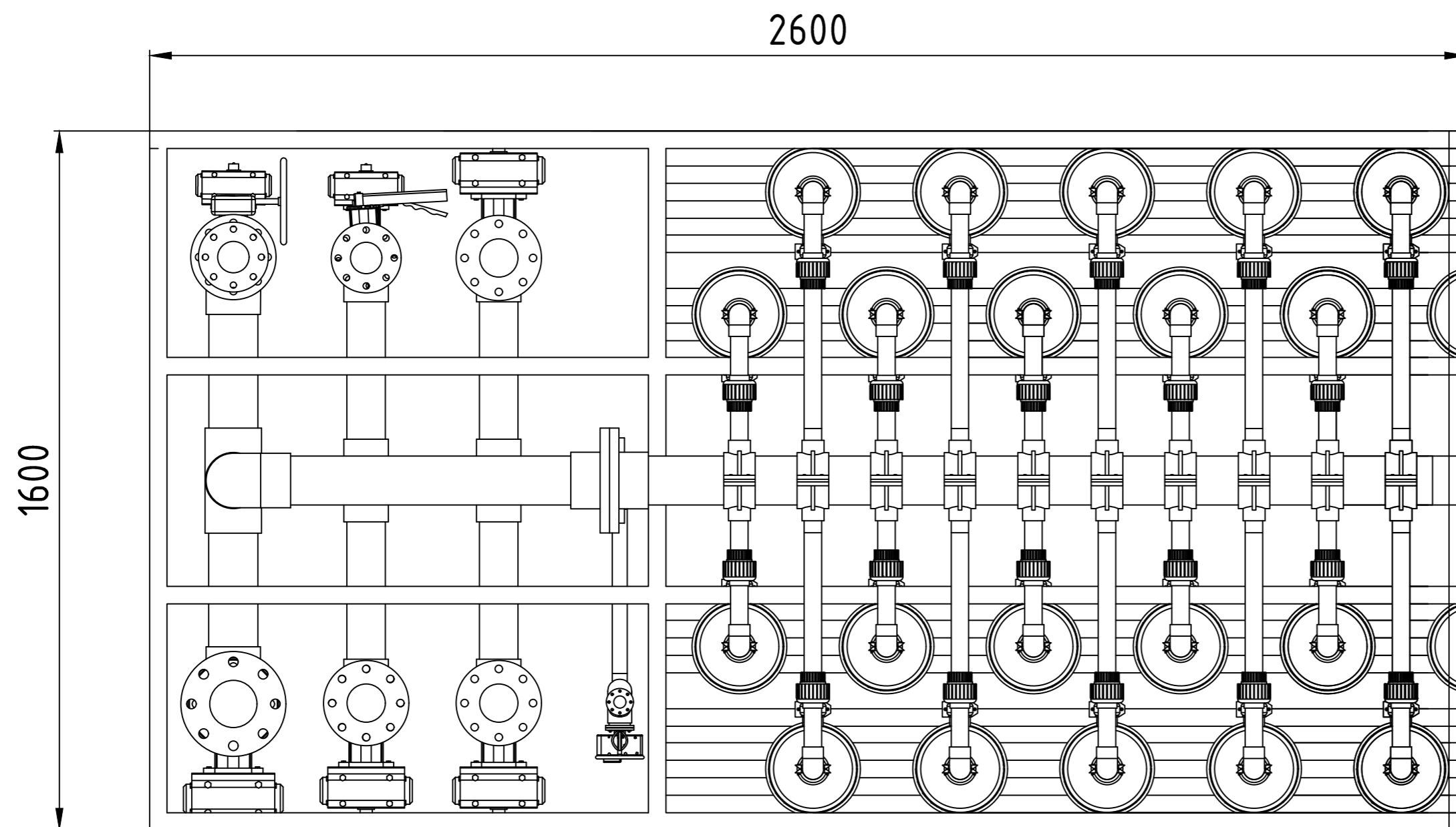
Вид сверху
