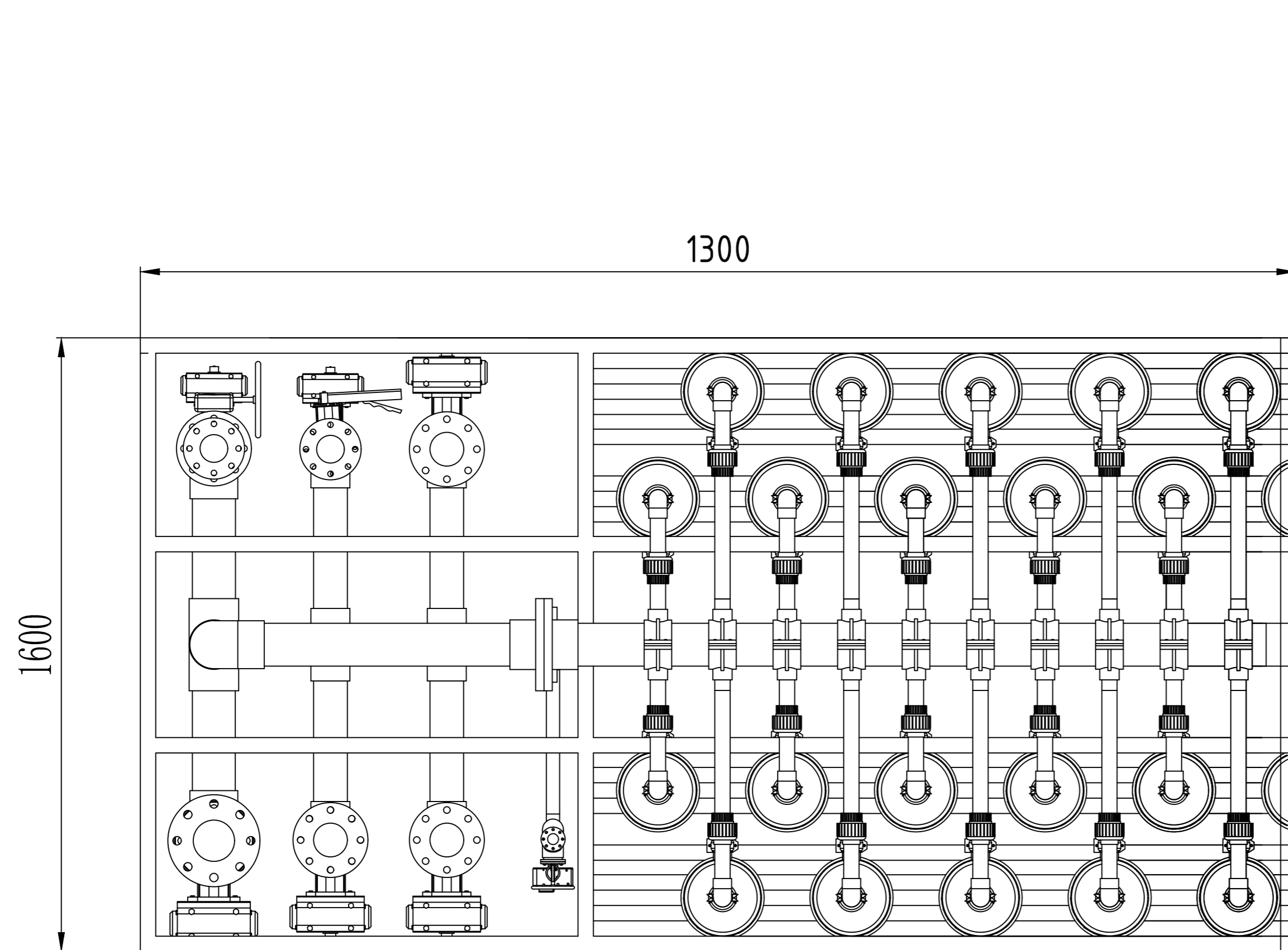
Вид сверху
