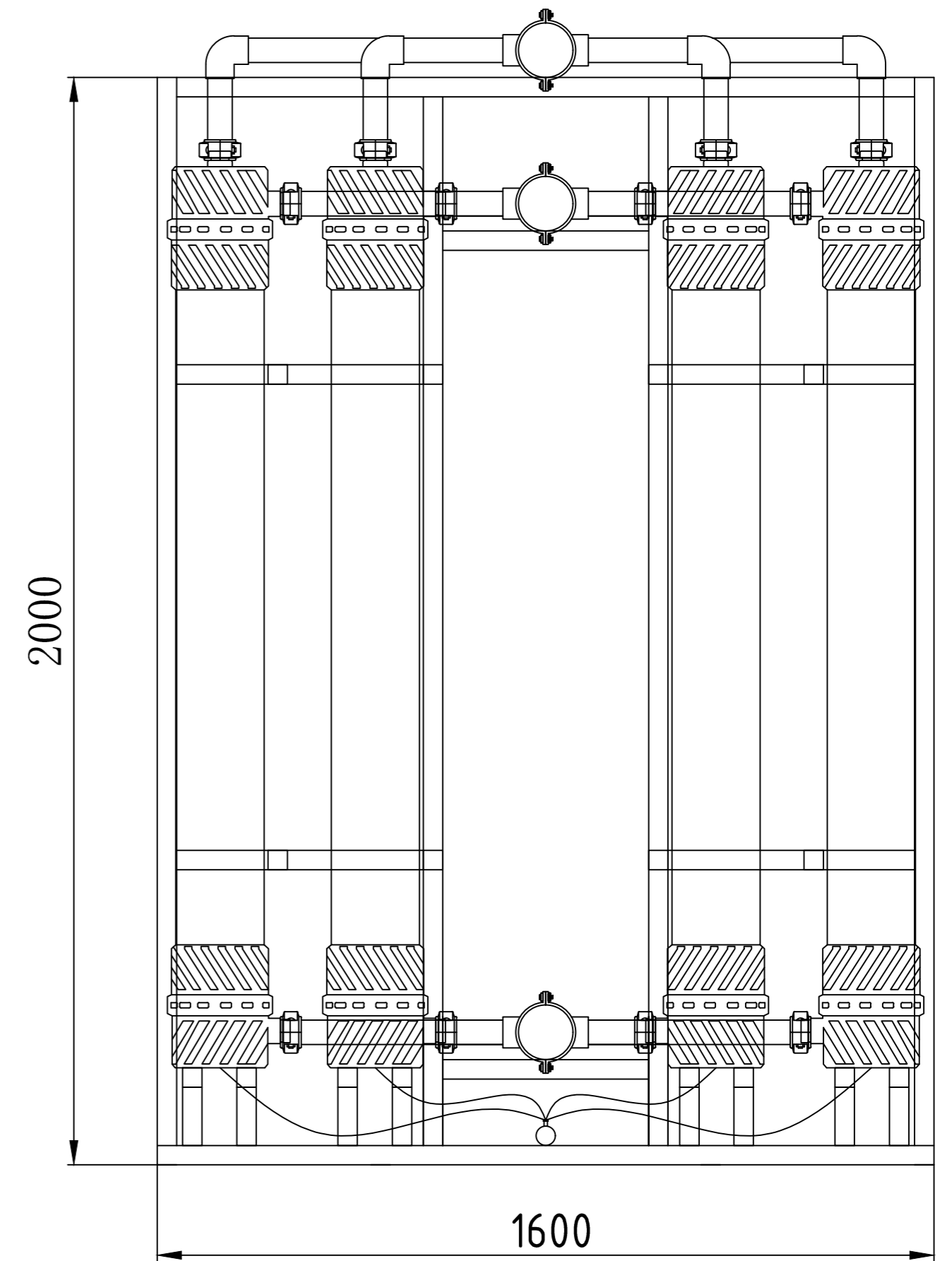
Вид слева
